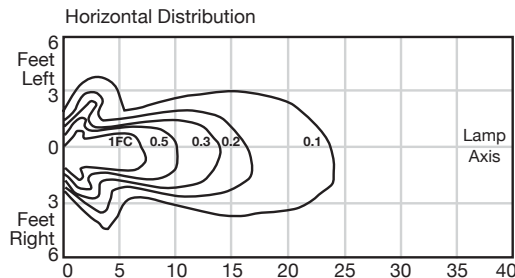
6V, 5.4W Tungsten Wedge Base Lamp (ANSI 939)
